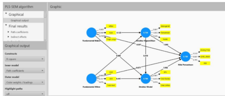
Gambar 3. Graphic Setelah Olah Data
