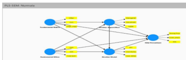
Gambar 2. PLS-SEM Olah Data
