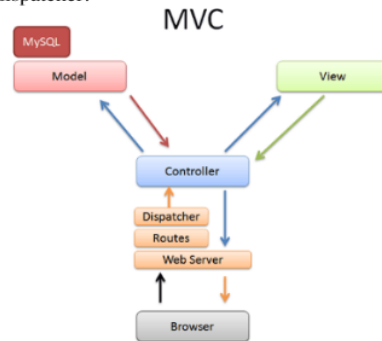
Gambar 1. Ilustrasi MVC dari Framework Codeigniter
