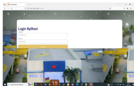
Gambar 2. Menu Login
