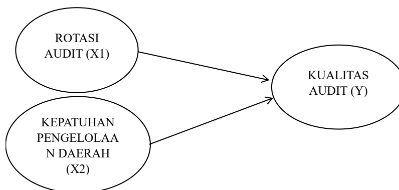
Gambar 1. Kerangka Pemikiran
