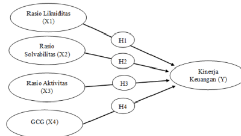
Gambar 2.2 Kerangka Konseptual
