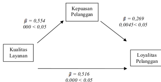
Gambar 6. Model Regresi dengan Mediator
