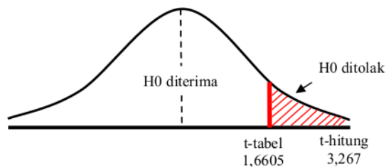
Gambar 4 Kurva Pengambilan Keputusan uji t (x-y)
