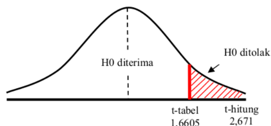
Gambar 5. Kurva Pengambilan Keputusan uji t (x-y)
