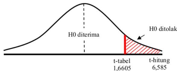
Gambar 3. Kurva Pengambilan Keputusan uji t (x-m)
