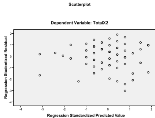
Gambar 2. Grafik Heteroskedastisitas ( Y = a + b_1X_1 + e )
